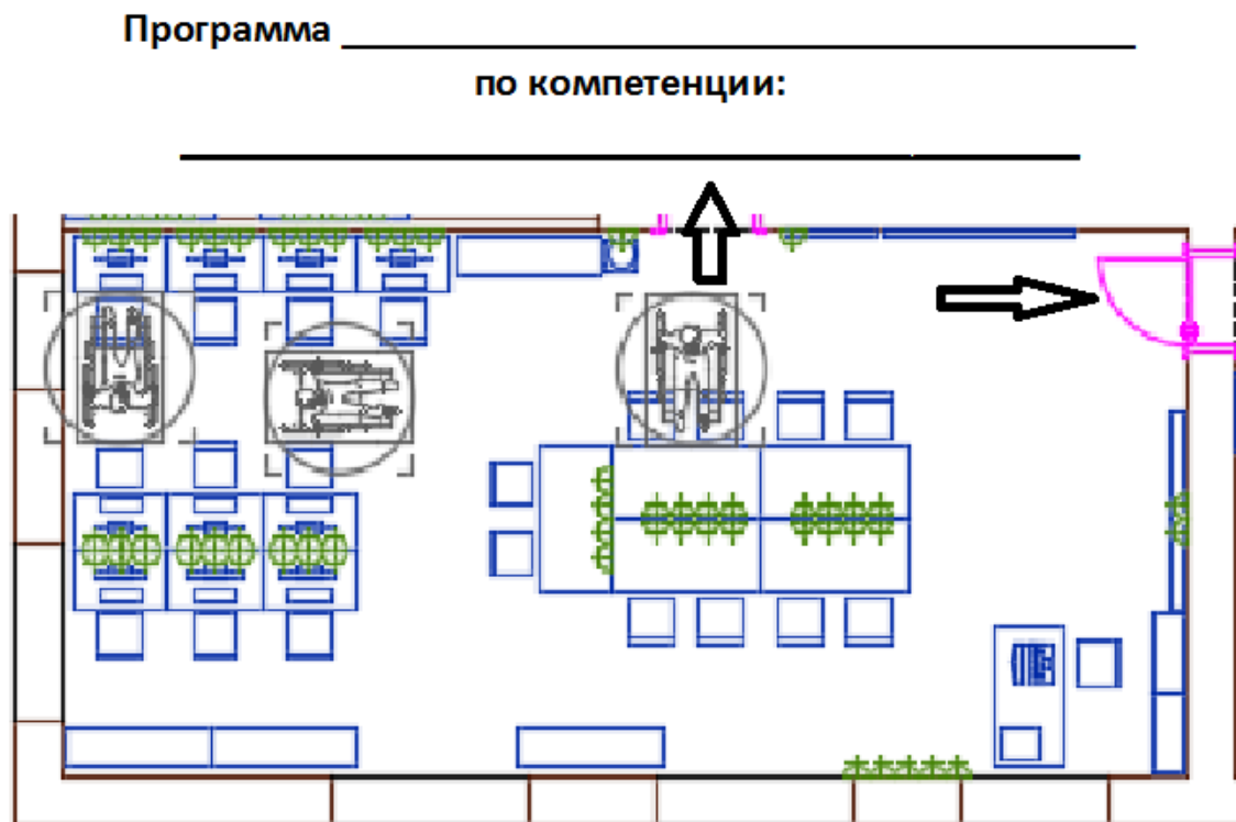
Рисунок 2 – План застройки
